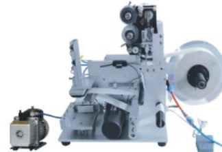
MT-60C Flat label machine with coding 平面貼標機帶打碼機
