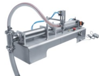
GC-A Semi-auto Liquid Filler 單頭氣動液體灌裝機
