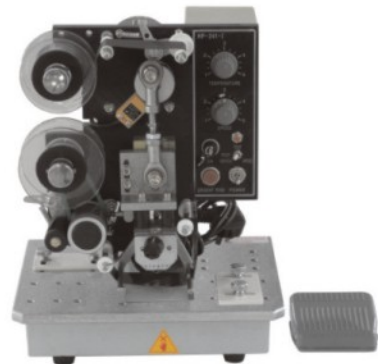
HP-241-I Hot Code Printer 電動熱打碼機
