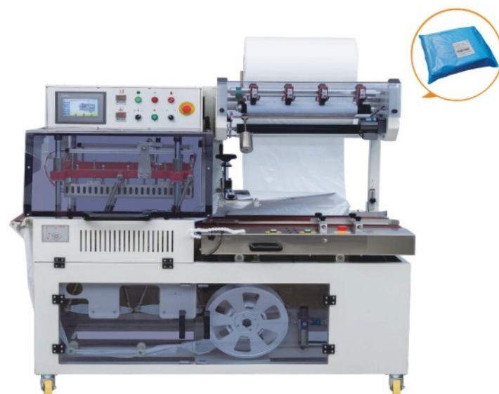
DQL5545PEG High Speed Automatic L Sealer For PE express bags 高速自動L型封切機（適用PE快遞袋）
