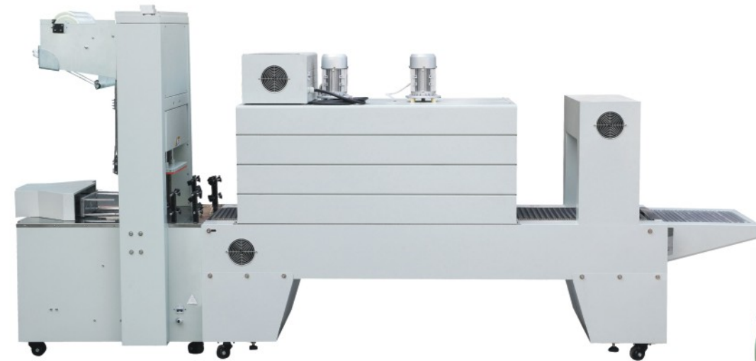
BZJ5038B(SEMI-AUTO SLEEVE WRAPPER)+BSE5040A(TUNNEL) 袖口式半自動包裝機+PE熱收縮包裝機
