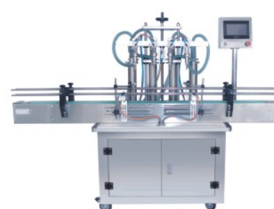
ZY Series Liquid Filler 直綫式液體灌裝機
