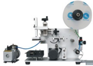
MT-60 Flat label machine 平面貼標機
